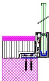
Garde-corps en tête de dalle
