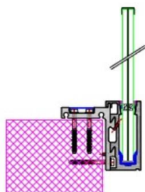
Garde-corps en tête de dalle
