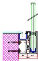
Garde-corps en tête de dalle avec gouttière
